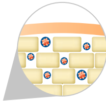
noreiz Wirkkomplex mit Thiocyanat
